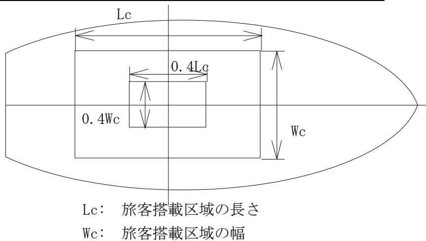
図 1 試験荷重の搭載位置
