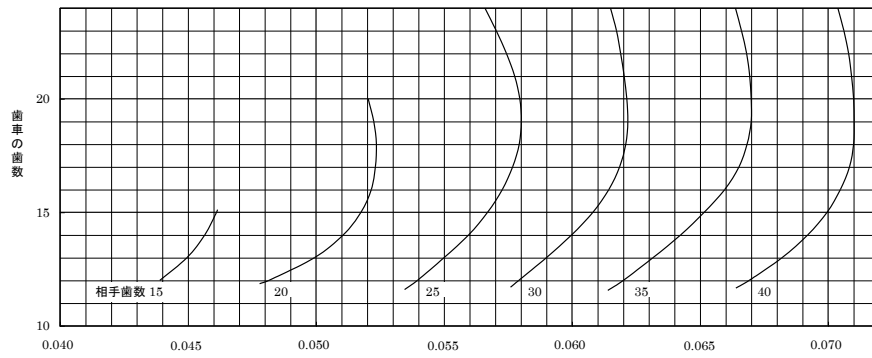
圧力角20° ネジレ角15° のマガリバカサ歯車の歯面強さの幾何係数 I
