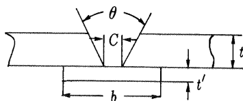
(c) V 型突合開先 (裏溶接不能の場合)
