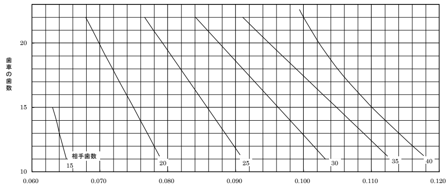
圧力角20° ネジレ角35° のマガリバカサ歯車の歯面強さの幾何係数 I
