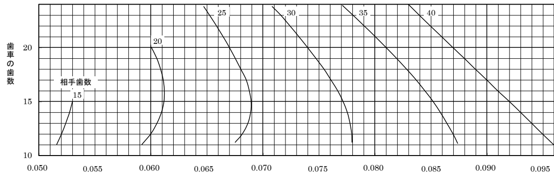
圧力角20° ネジレ角25° のマガリバカサ歯車の歯面強さの幾何係数 I
