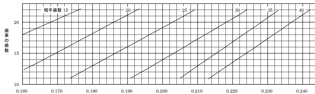
圧力角20° ネジレ角35° 軸角90° のマガリバカサ歯車の曲げ強さの幾何係数 J
