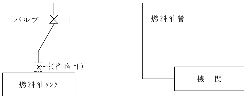
図35.3<3> 弁又はコックを燃料油タンク壁に連結させなくてよい場合 (e) タンクの頂部より低い位置に燃料油管が配置されない場合は、 弁又はコックを備え付けなくても差し支えない(図35.3<4>参照)。
