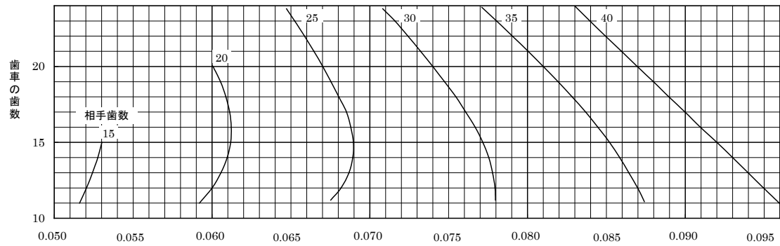
圧力角 20^\circ ネジレ角 25^\circ 軸角 90^\circ のマガリバカサ歯車の歯面強さの幾何係数 I
