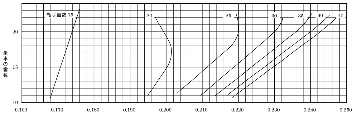
圧力角20° 軸角90° のスグバカサ歯車、ゼロール歯車の曲げ強さの幾何係数 J
