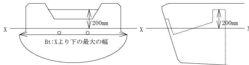
図1 モーターウエルを有するもの
