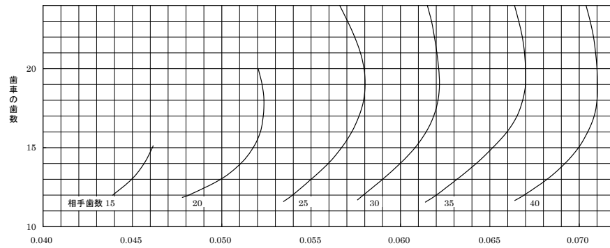
圧力角 20^\circ ネジレ角 15^\circ 軸角 90^\circ のマガリバカサ歯車の歯面強さの幾何係数 I
