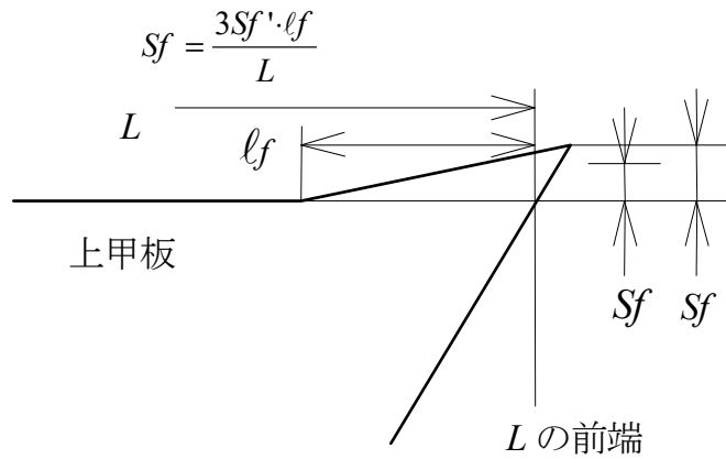
図7.1<2> 直線舷弧の Sf (2)
