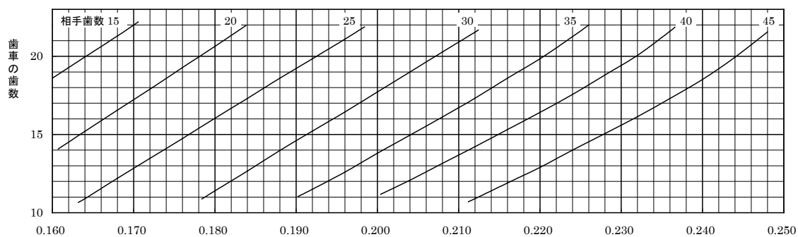
圧力角20° ネジレ角25° 軸角90° のマガリバカサ歯車の曲げ強さの幾何係数 J
