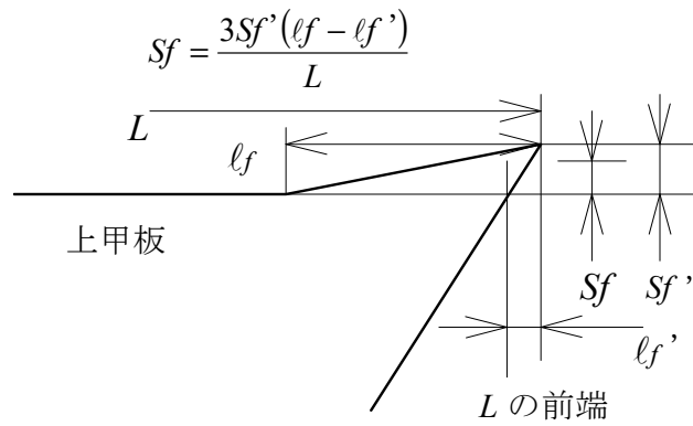
図7.1<1> 直線舷弧の Sf (1)
