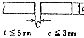
(a) I 型突合開先
