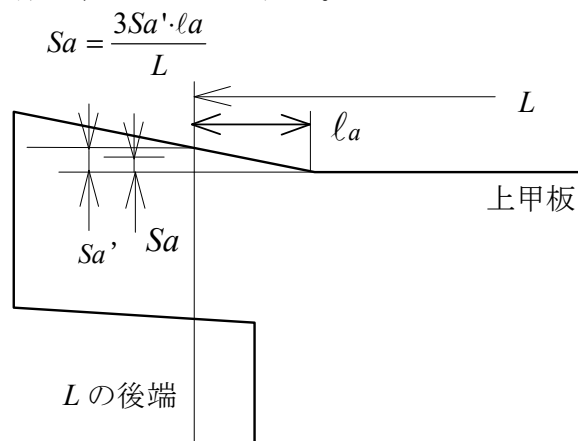
図7.1<3> 直線舷弧の Sa
