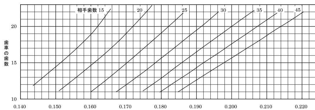
圧力角20° ネジレ角15° 軸角90° のマガリバカサ歯車の曲げ強さの幾何係数 J
