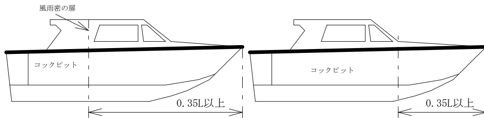
図 7. 3<2> コックピットの前端の位置
