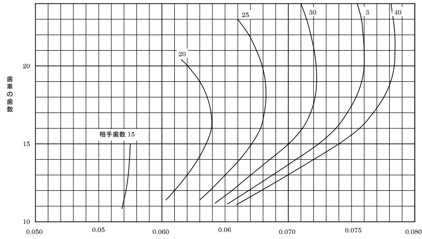
圧力角 20^\circ 軸角 90^\circ のスグバカサ歯車、ゼロール歯車の歯面強さの幾何係数 I
