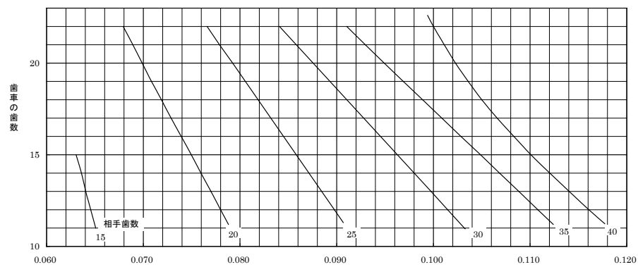
圧力角 20^\circ ネジレ角 35^\circ 軸角 90^\circ のマガリバカサ歯車の歯面強さの幾何係数 I
