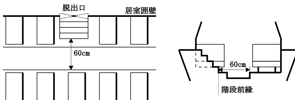
図 75.1<9> 客室甲板に段があるときの階段の前縁の取り扱い
