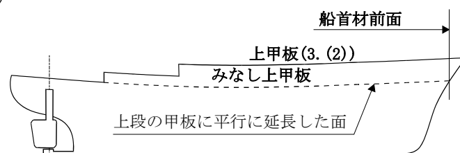
図6 2-2(2)の上甲板を有する場合
