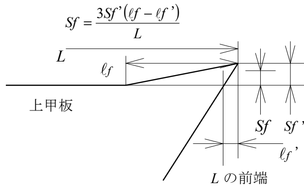
図7.1<1> 直線舷弧の Sf (1)
