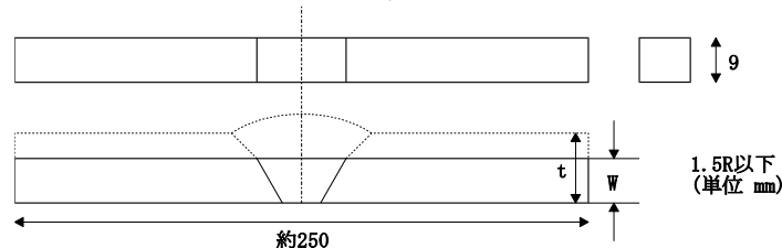
側曲げ試験片
