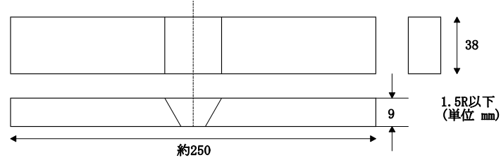
図4 溶接部の曲げ試験片
