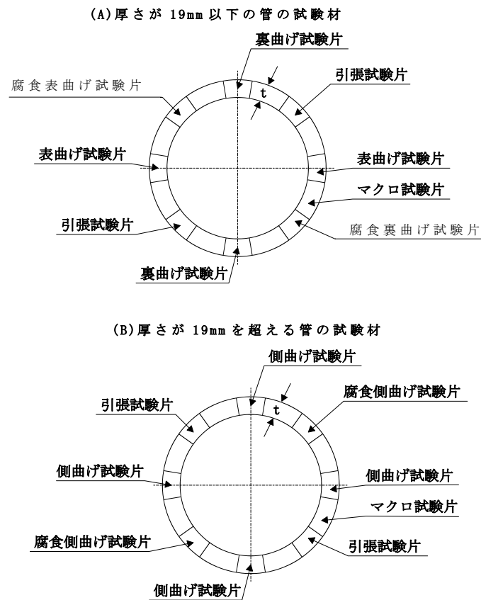
図 2 管の溶接施工方法試験試験材
