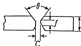
(e) X 型突合開先
