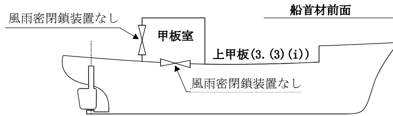
図9 2-2(3)(i)の上甲板を有する場合
