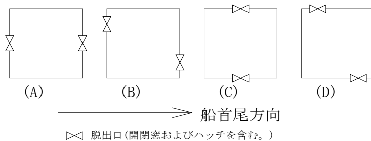
図81.1<1> 望ましい脱出口の配置の例
