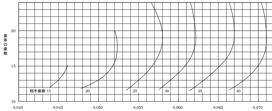
圧力角20° ネジレ角15° 軸角90° のマガリバカサ歯車の歯面強さの幾何係数 I
