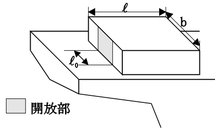
図81.1<5> 脱出設備の要件に適合しているとみなす開口の例
