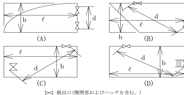
図 81.1<2> 脱出口を d \geq \frac{2}{3}b とすること。 (A) d \geq \frac{2}{3}l , (B) d \geq \frac{2}{3}l , (C) d \geq \frac{2}{3}l , (D) d \geq \frac{2}{3}l
