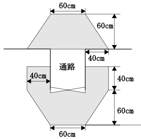
図 75. 1<3> 脱出口の前後に天井まで壁を設けた場合
