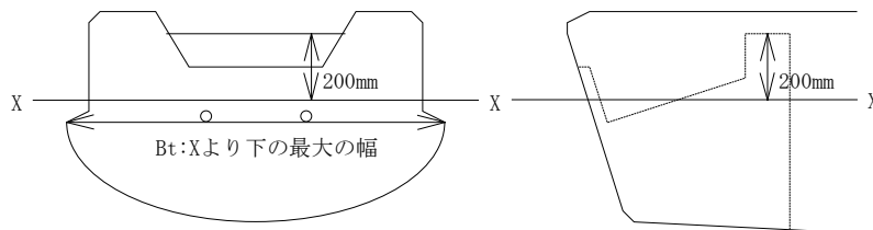
図1 モーターウエルを有するもの
