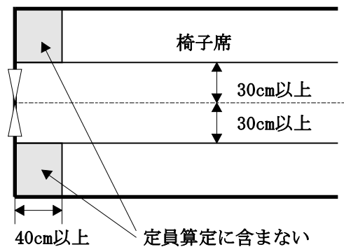
図 75.1<5> 〇部は定員算定場所としてはならないが、椅子席自体は設けてもよい。
