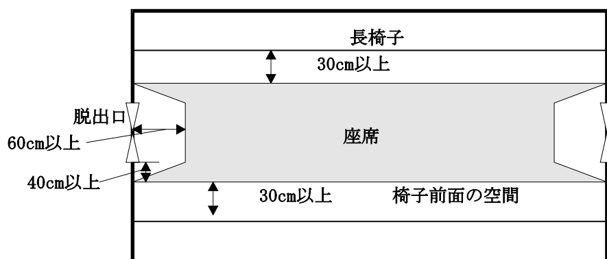
図 75.1<6> 居室を座席とし、周囲に長椅子を配置した場合、特に通路をとらず、脱出口周辺及び椅子の前面の空間30cmを除いた〇を座席定員の算定場所としてよい。
