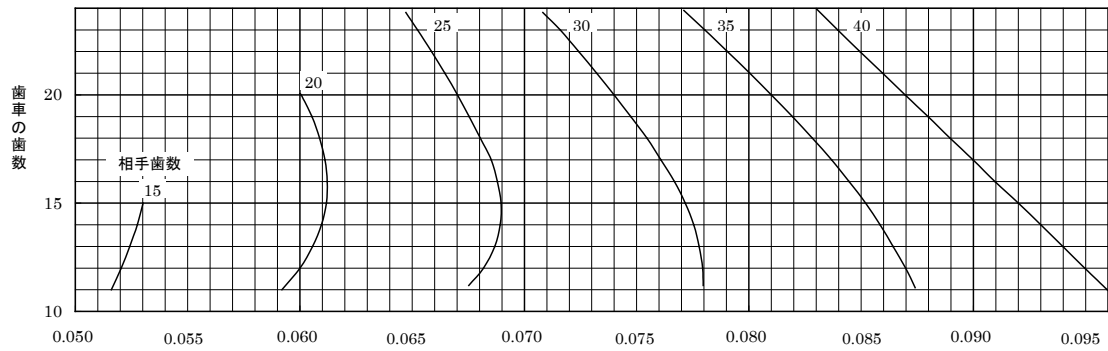
圧力角20° ネジレ角25° 軸角90° のマガリバカサ歯車の歯面強さの幾何係数 I
