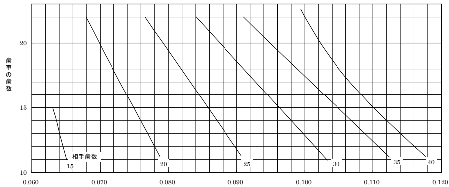
圧力角20° ネジレ角35° 軸角90° のマガリバカサ歯車の歯面強さの幾何係数 I
