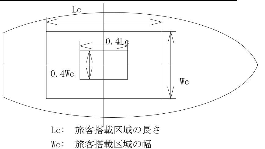
図 1 試験荷重の搭載位置
