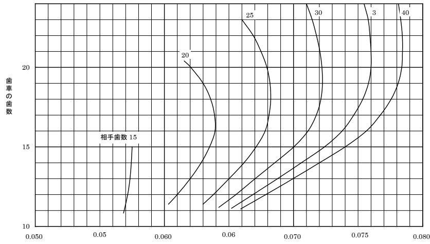
圧力角20° 軸角90° のスグバカサ歯車、ゼロール歯車の歯面強さの幾何係数 I
