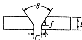
(b) V 型突合開先
