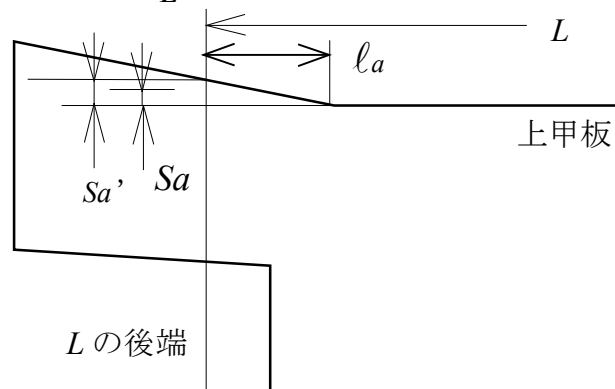
図7.1<3> 直線舷弧の Sa
