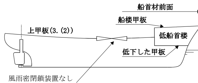
図5 2-2(3)(i)の上甲板を有する場合
