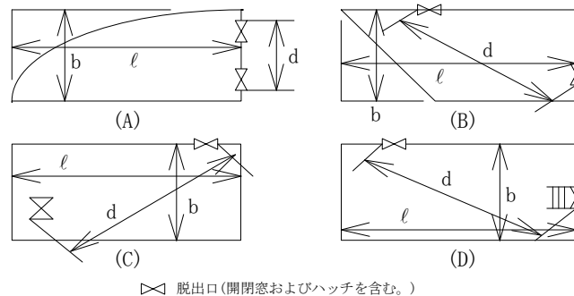
図 81.1<2> (d \geq \frac{2}{3}l, \text{脱出口を} d \geq \frac{2}{3}b \text{とすること。}) の配置の例
