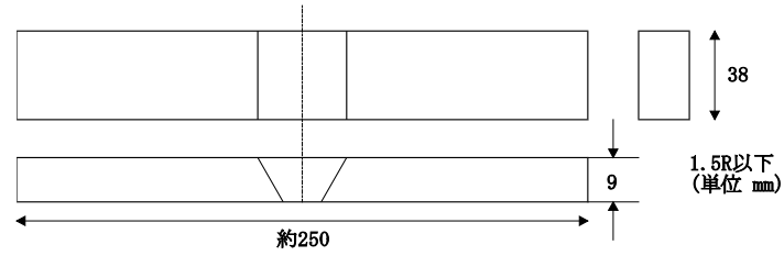
図4 溶接部の曲げ試験片
