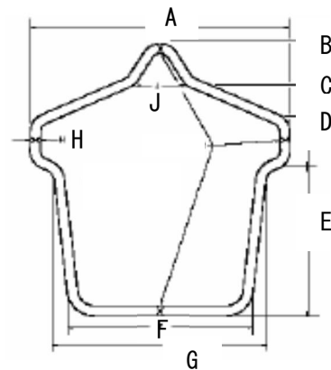
垂直強度試験用型
