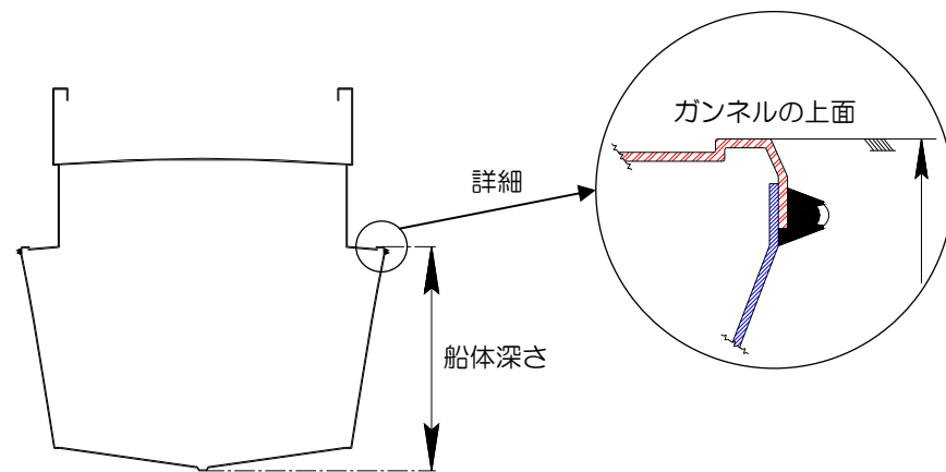
(a) 通常のガンネル
